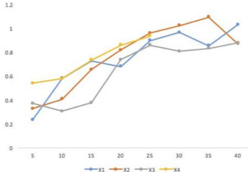
図 6 X 軸断面それぞれにおける深さとコーン指数の関係
